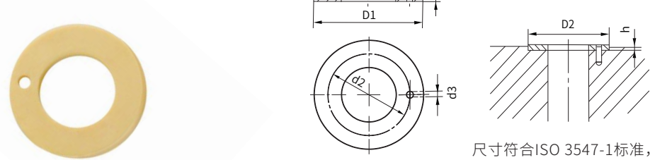
止推垫圈- T型(mm)
